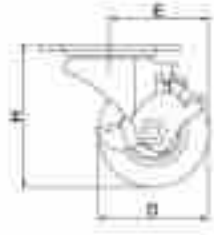
回转制动器
