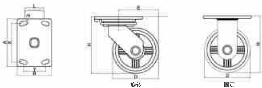
外形图 |
