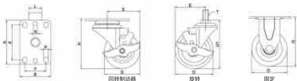
外形图
