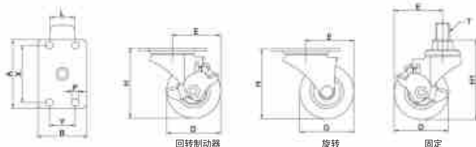
回转制动器
