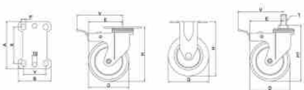
外形图
