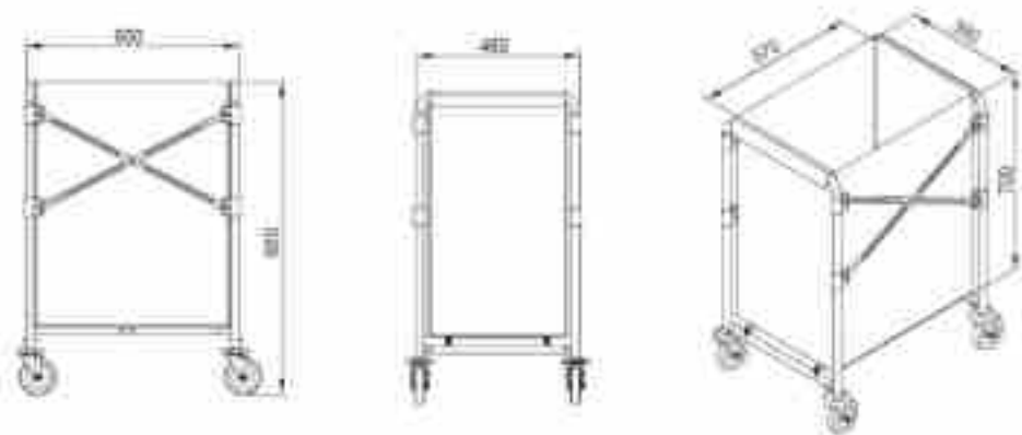
外形图
