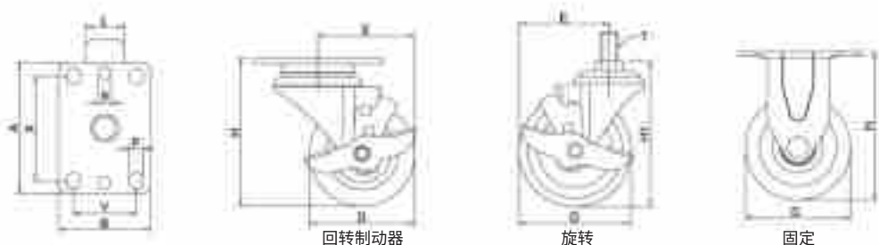
外形图 |
